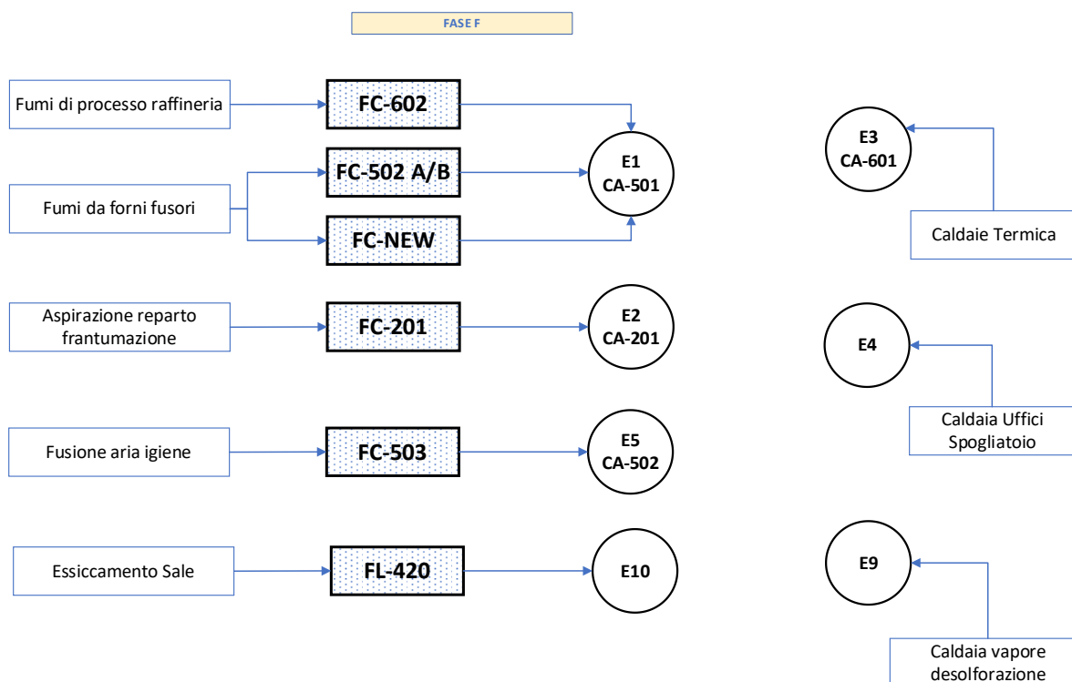
Figura B.7 Schema di flusso Fase “F” Emissioni in atmosfera
