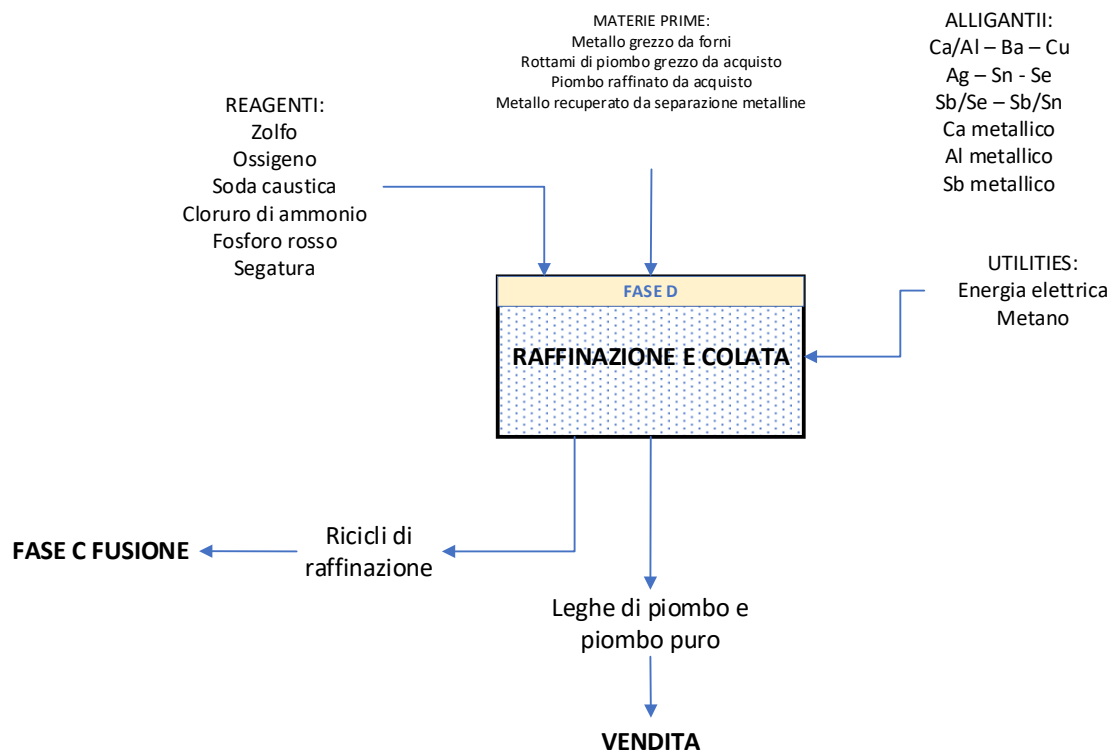
Figura B.5 Schema di flusso Fase “D” Raffinazione e Colata
