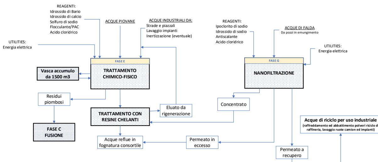
Figura B.6 Schema di flusso Fase "E" Trattamento acque industriali e Fase "G" trattamento acque di falda
