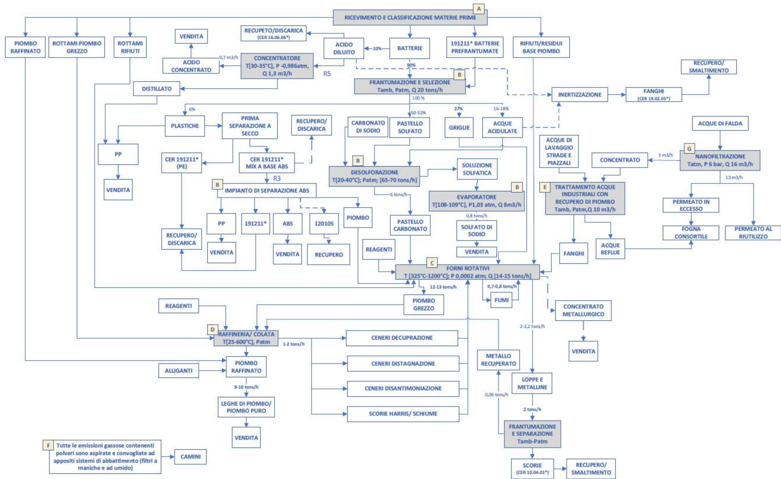
Figura B.1 Schema di flusso dell'intero ciclo
