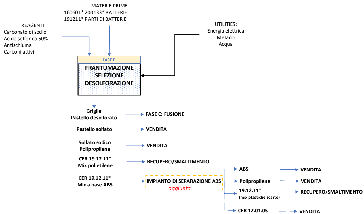
Figura B.3 Schema di flusso Fase “B” Frantumazione e Desolfurazione
