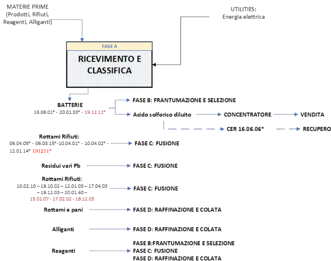
Figura B.2 Schema di flusso Fase "A" Ricevimento e classificazione materie in ingresso
