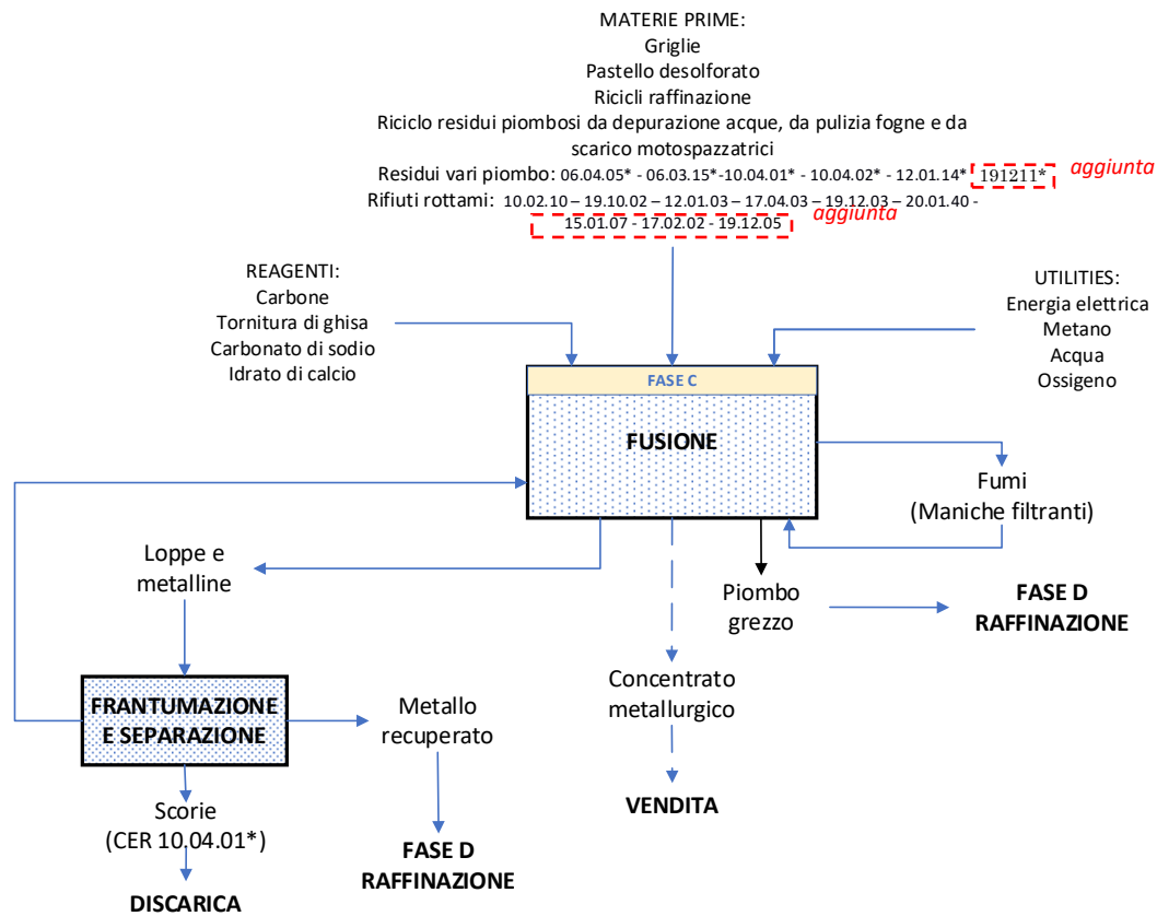
Figura B.4 Schema di flusso Fase "C" Fusione
